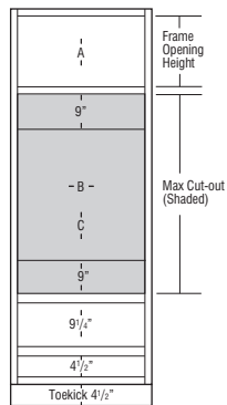
OCS_24DDN
