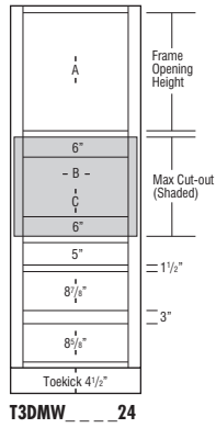
T3DMW _ _ _ 24
