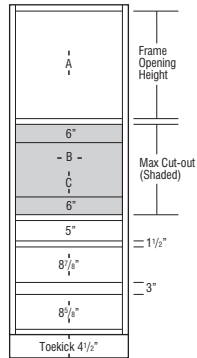
T3DMW _ _ _ 24N
