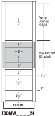
T3DMW _ _ _ _ 24
