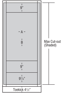
OCD_6624DD
