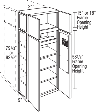
UOCDZ24849AEL/AER UOCDZ24879AEL/AER
