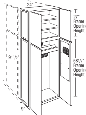
UOCDZ24969EL/AER
