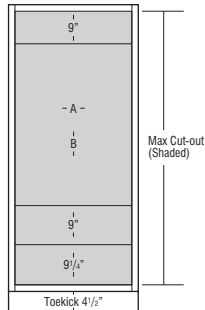
OCD_6624DDN
